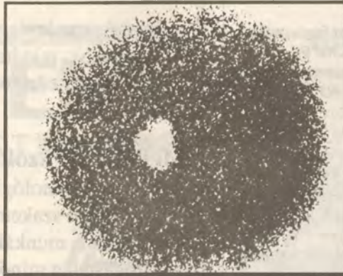
A Plútó legjobb képének százsoros nagyítása egy 155 centiméteres lemeztől. A hold az az enyhe, jobbra felmutató kidudorodás, mely a bolygó képeinek felső részéből indul ki. (A Mercury Magazine 1979. január-februári számából, © Astronomical Society of the Pacific.)
